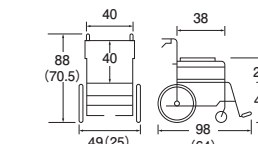
( )は折りたたみ時 単位: cm
