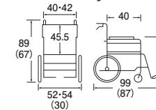
( )は折りたたみ時 単位: cm
