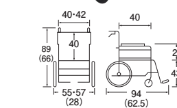
( )は折りたたみ時 単位: cm
