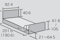
スリムボード83cm幅 (単位: cm)
