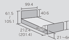
樹脂ボード91cm幅 (単位: cm)
