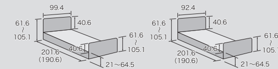
スリムボード91cm幅 (単位: cm)
