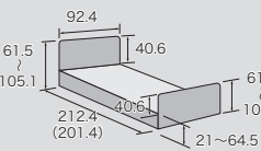
樹脂ボード83cm幅 (単位: cm)
